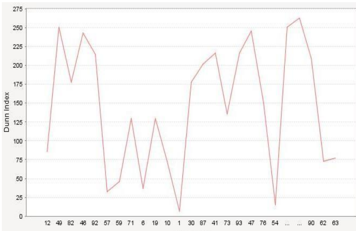
Fig. 4 Dunn Index
